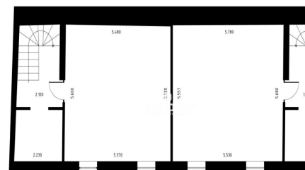
ПЛАН ПОДВАЛА
