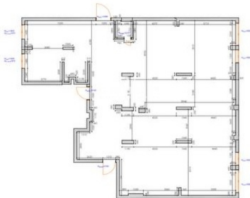
Обмерный план, М 1:100
