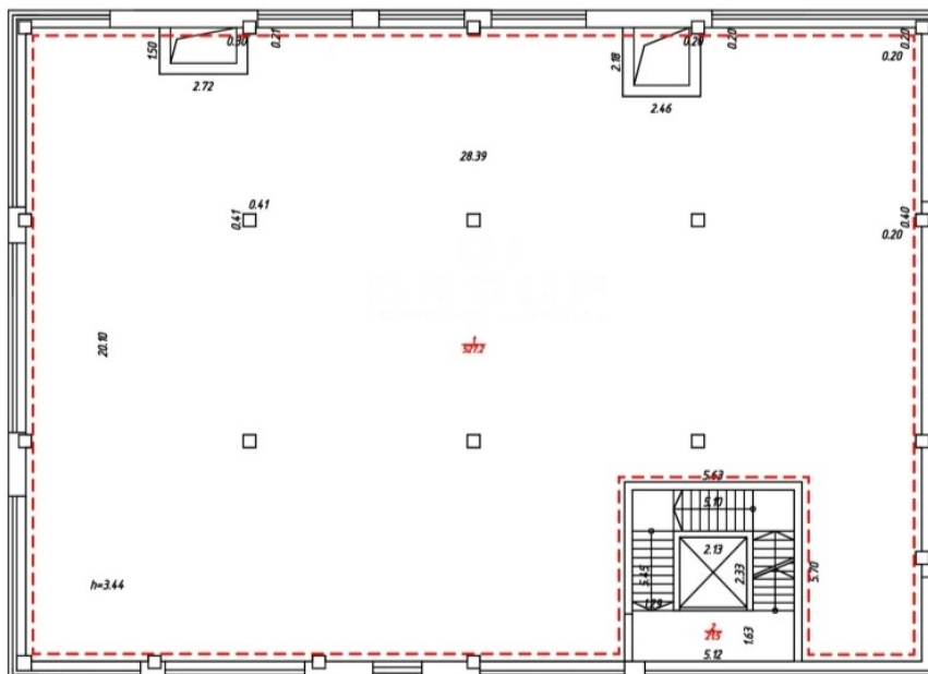
ТЕХНИЧЕСКИЙ ПЛАН ЗДАНИЯ ПЛАН ЭТАЖА ЧАСТИ ЭТАЖА 2 ЭТАЖ
