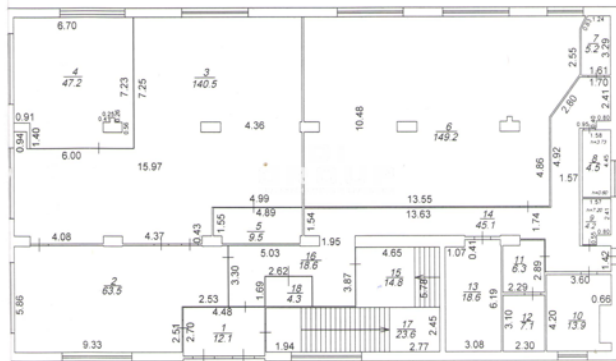
план 1 этажа
