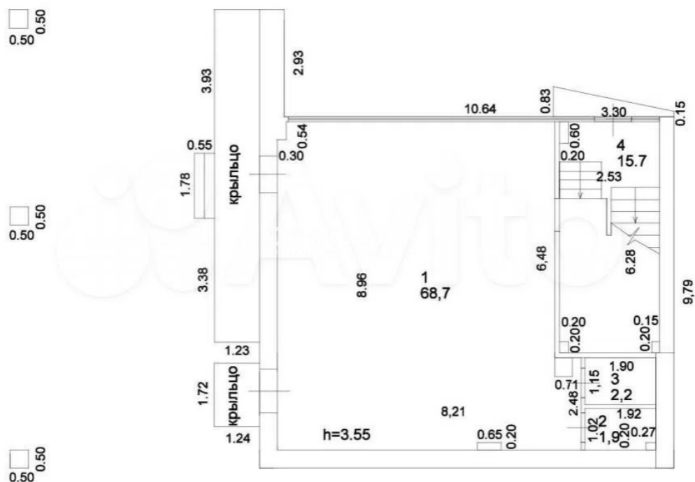
План 1 этажа
