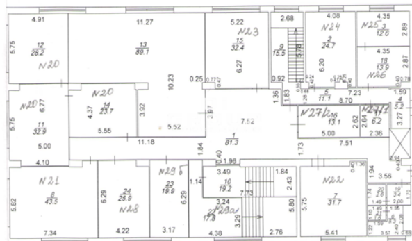
план 2 этажа
