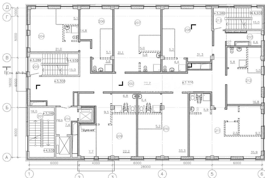
План 2—3 этажей
