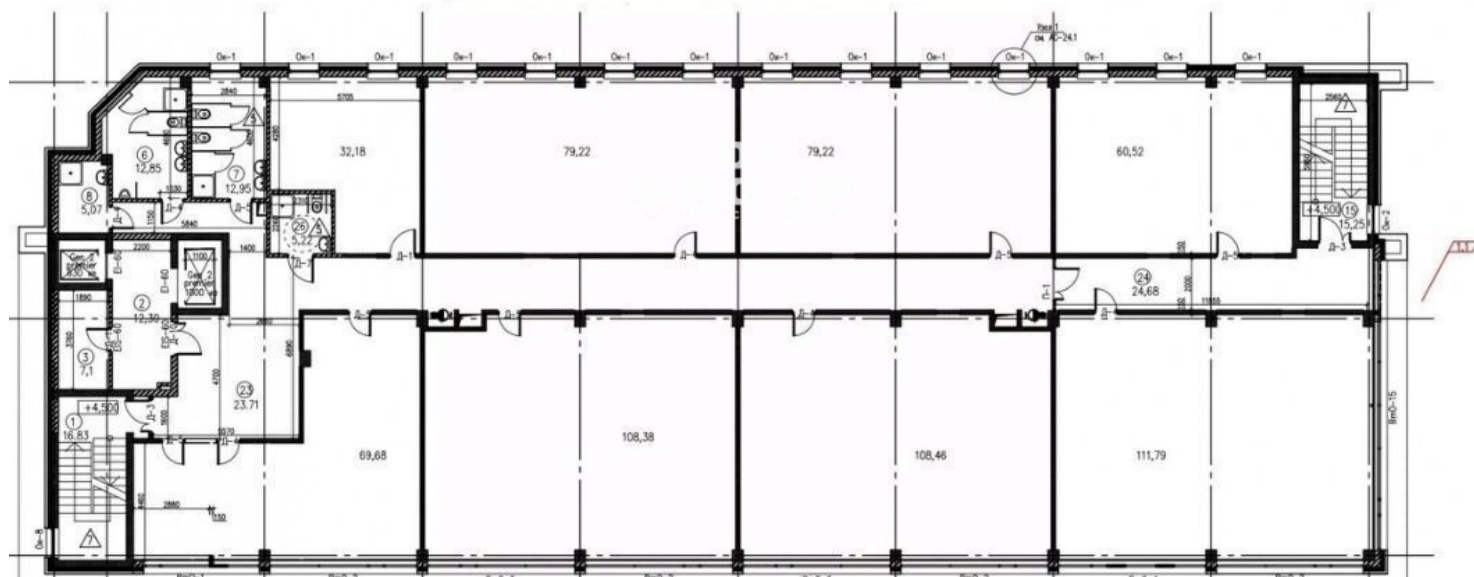
Отделочный план 3-го этажа на отметке 8,100
