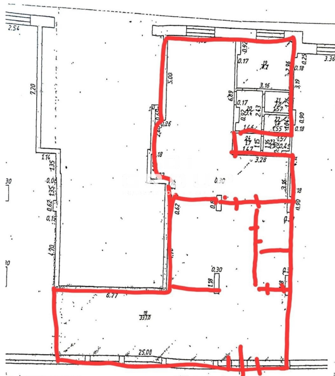
ПОЭТАЖНЫЙ ПЛАН
