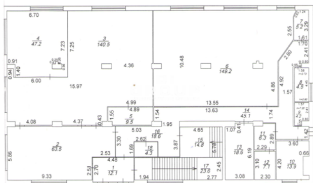
план 1 этажа
