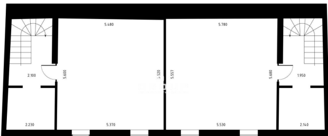
ПЛАН ПОДВАЛА
