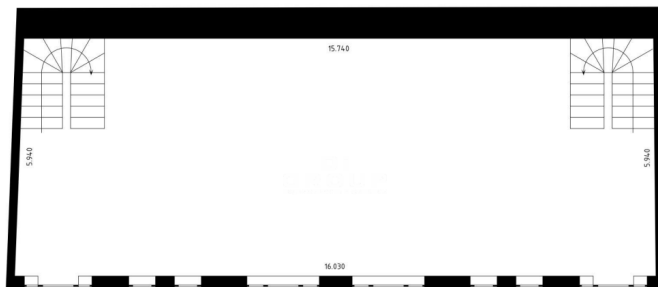
ПЛАН ВТОРОГО ЭТАЖА
