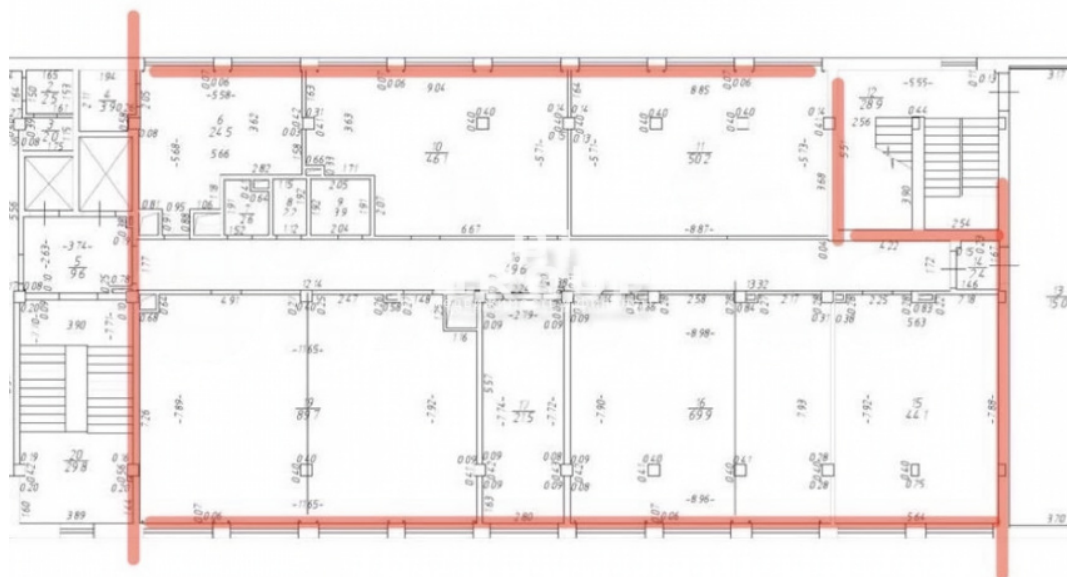
План 6 этажа
